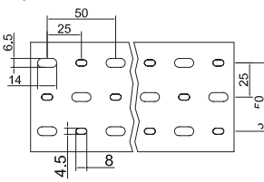
150宽为5排底孔
