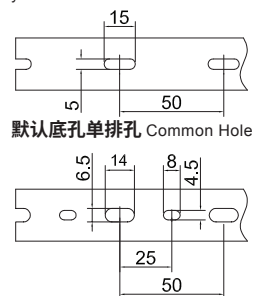
可定制大小孔/EU Hole of DIN
